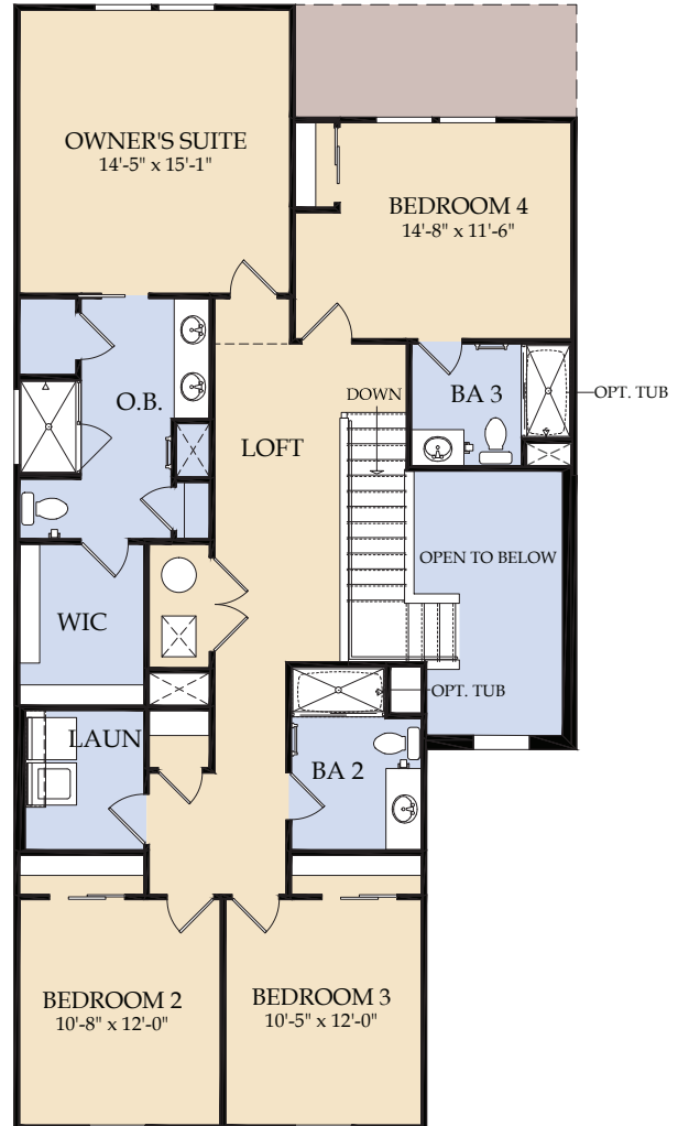
Segundo andar
