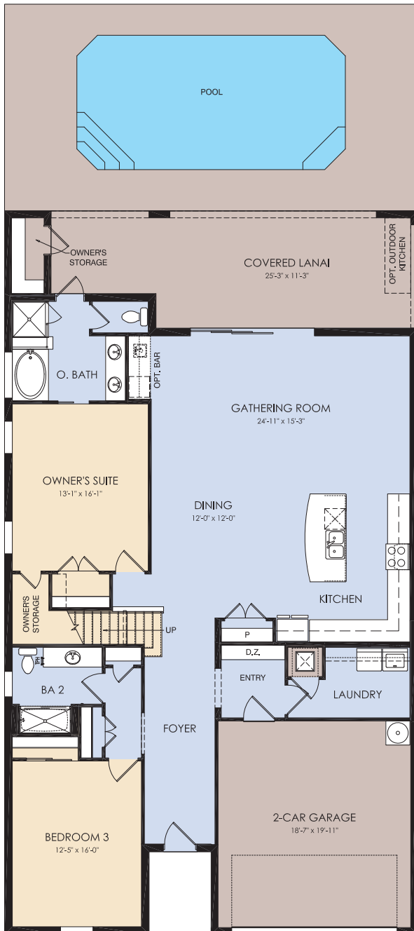
Primeiro andar
